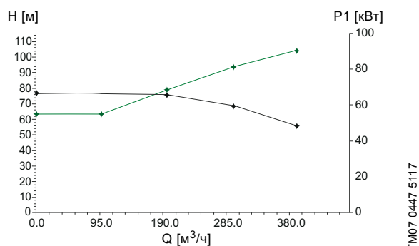
Рис. 83 Результаты измерений для испытываемого насоса
