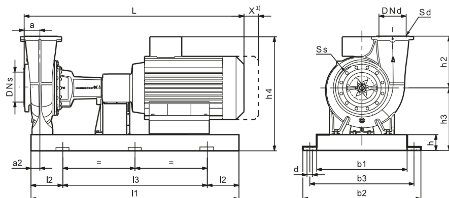
Рама- основание EN/ISO, тангенциаль- ный отвод
