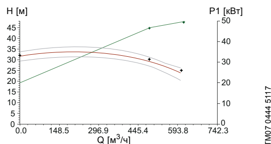
Рис. 82 Расчет значений на рис. 81 произведен для стандартной частоты с целью сравнения с эталонной эксплуатационной характеристикой
