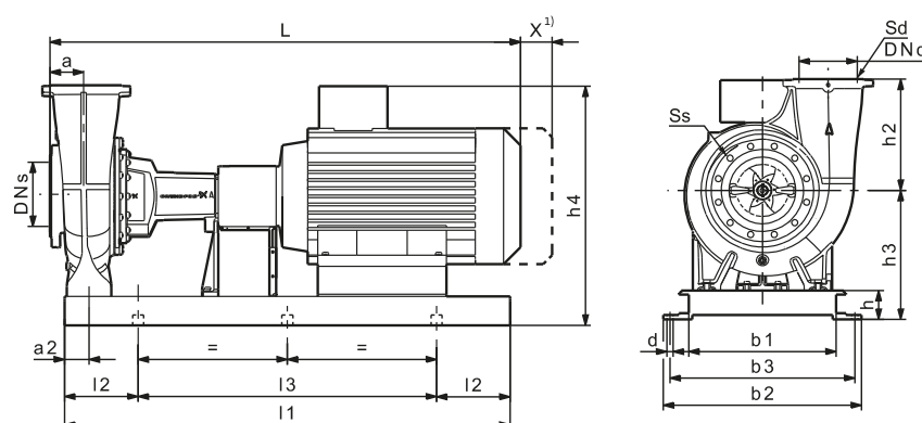
С-образная рама- основание, тангенциаль- ный отвод
