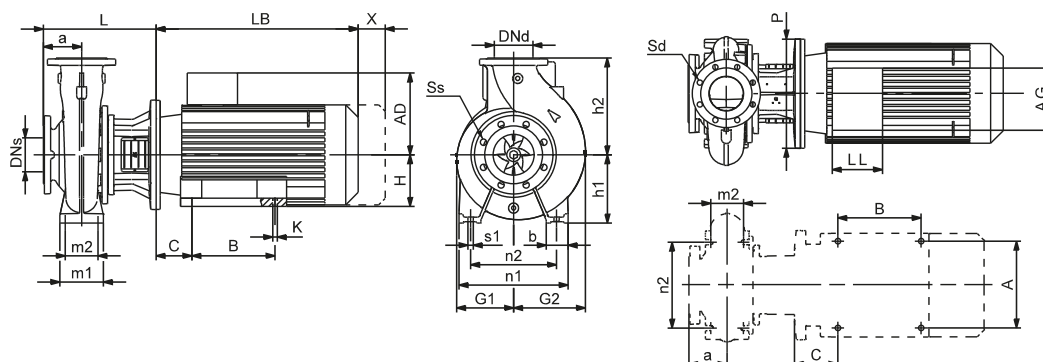
Исполнение C1, радиальный отвод
