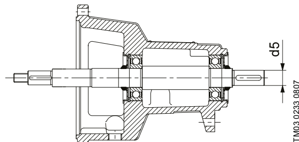
Рис. 23 Подшипниковый узел и вал
