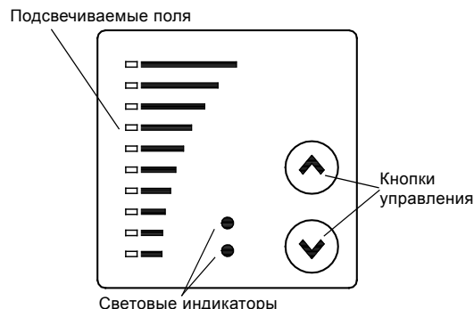
Рис. 69 Панель управления для 2-полюсных (15-22 кВт) и 4-полюсных (11 - 18,5 кВт) электродвигателей
