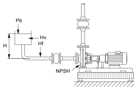
Рис. 48 Высота всасывания воды при отрицательном значении H_{всac}
