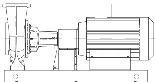
Рис. 86 Насос NKG с С-образной рамой-основанием
