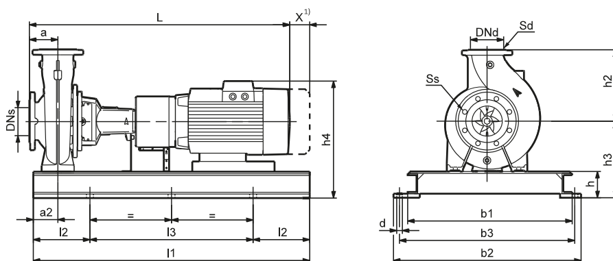
С-образная рама- основание, радиальный отвод
