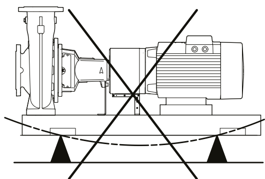
Рис. 51 Неправильная установка
