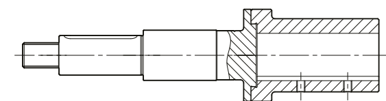
Рис. 28 2-секционный вал насоса NBG
