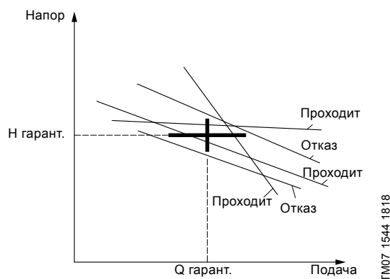
Рис. 75 Кривые насоса, которые проходят через допустимую область гарантируемой точки или не попадают в нее
