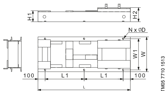
Рис. 92 С-образная рама-основание с 6 установочными отверстиями
