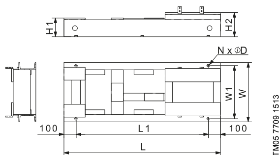
Рис. 91 С-образная рама-основание с 4 установочными отверстиями
