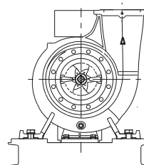
Рис. 33 Схематичное изображение насоса NKG в сборе на С-образной раме-основании
