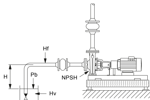
Рис. 47 Высота всасывания воды при положительном значении H_{всac}
