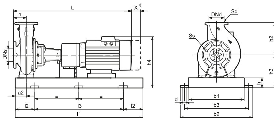
Рама- основание EN/ISO, радиальный отвод
