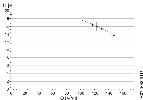
Рис. 74 Для определения одной гарантируемой точки используются результаты замеров на пяти контрольных точках
