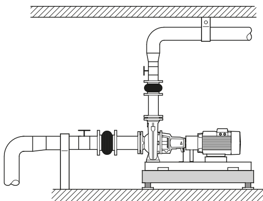
Рис. 56 Монтаж трубопровода
