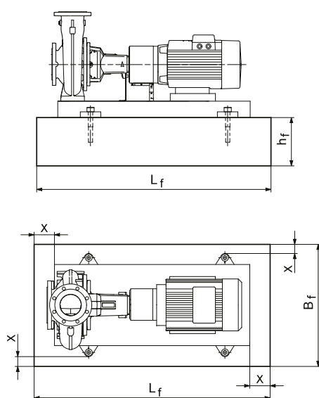
Рис. 49 Фундамент, X = мин. 100 мм
