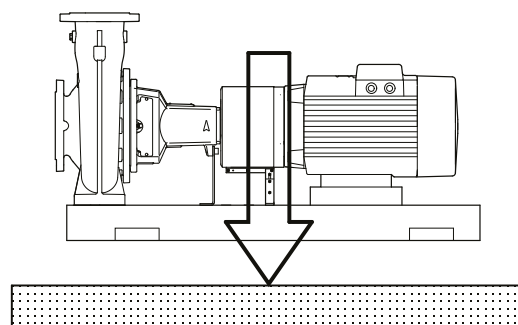
Рис. 50 Правильная установка
