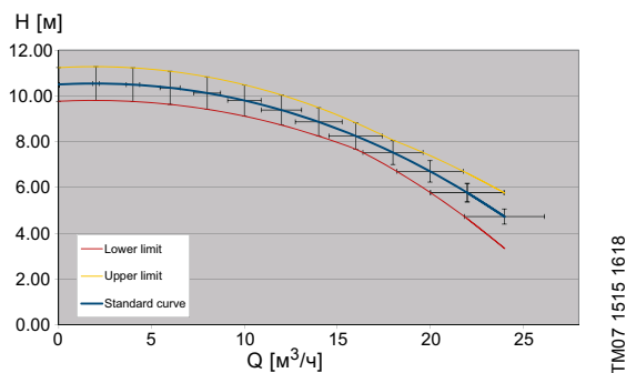
Рис. 80 Кривая Q-H с пересечениями допусков по всему диапазону рабочих характеристик
