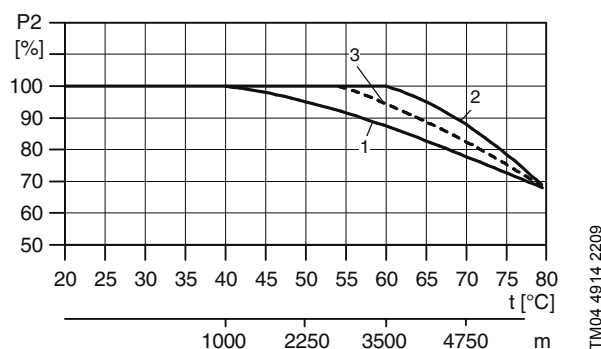
Рис. 38 Мощность двигателя в зависимости от температуры / высоты над уровнем моря
