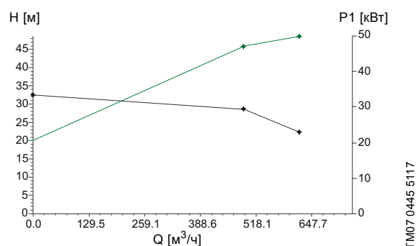
Рис. 81 Результаты измерений для испытываемого насоса
