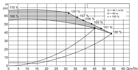
Рис. 64 Пример расширенного диапазона производительности до 110 % в рамках рабочего диапазона
