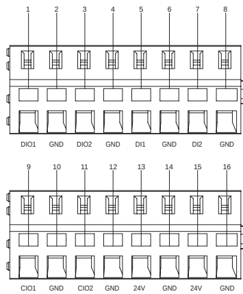
Рис. 120 Клеммы входов/выходов
