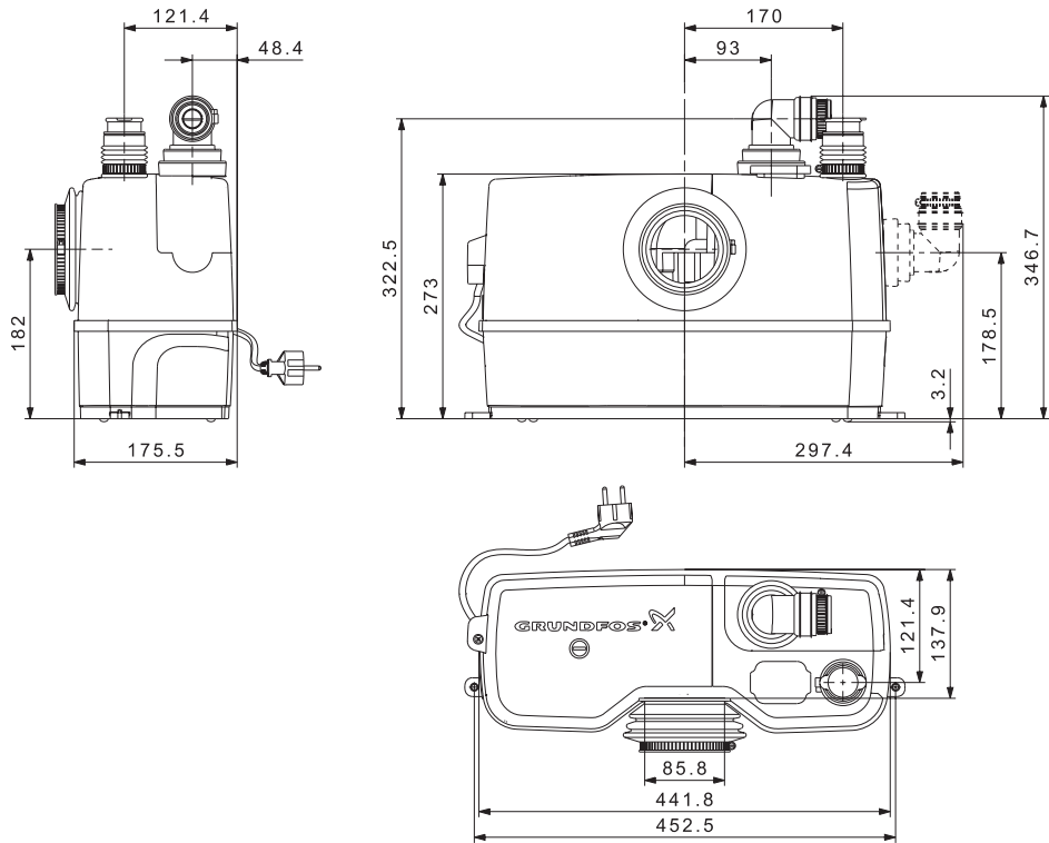
Рис. 57 Габаритные размеры, SOLOLIFT2 WC-1
