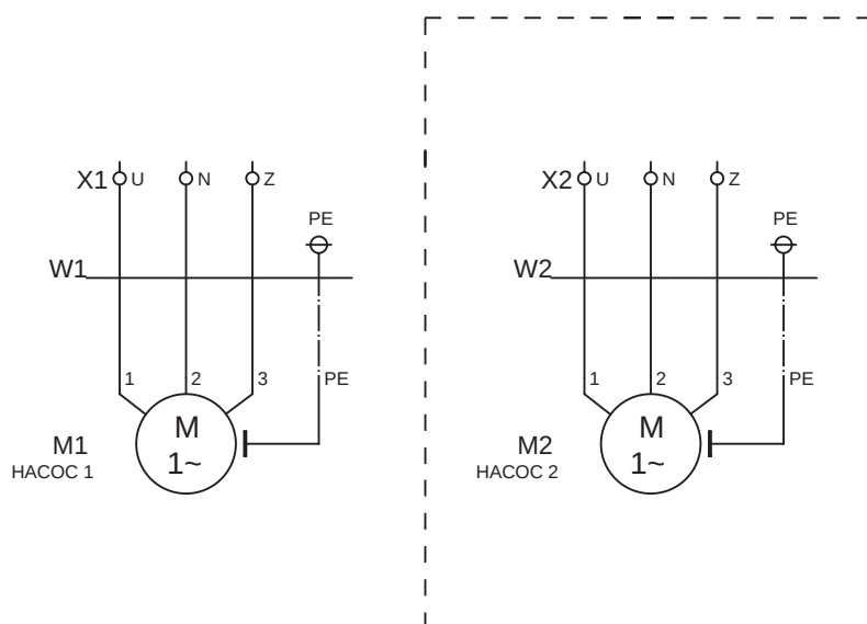
Рис. 123 Подключение однофазных насосов без конденсаторов (конденсаторы в составе шкафа)
