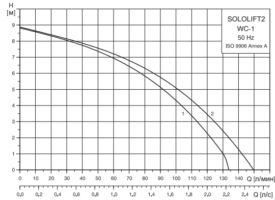
Рис. 56 Кривые характеристик
