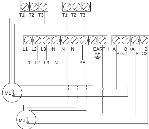
Рис. 119 Трехфазное подключение для двух насосов
