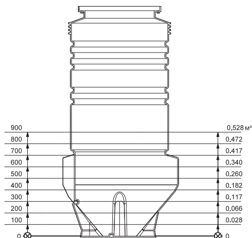
Рис. 140 Полезный объем относительно уровня, PS.R.10
