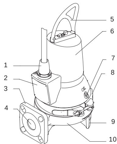
Рис. 42 Детализация насоса SEG
