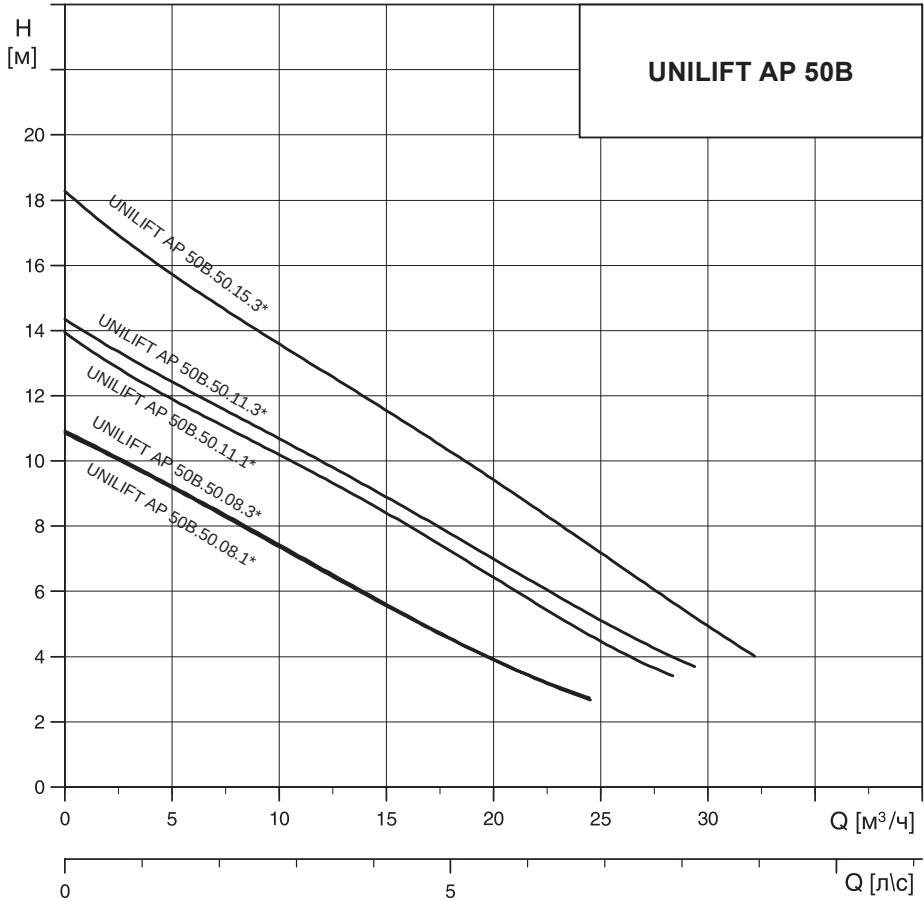
Рис. 30 Кривые характеристик
