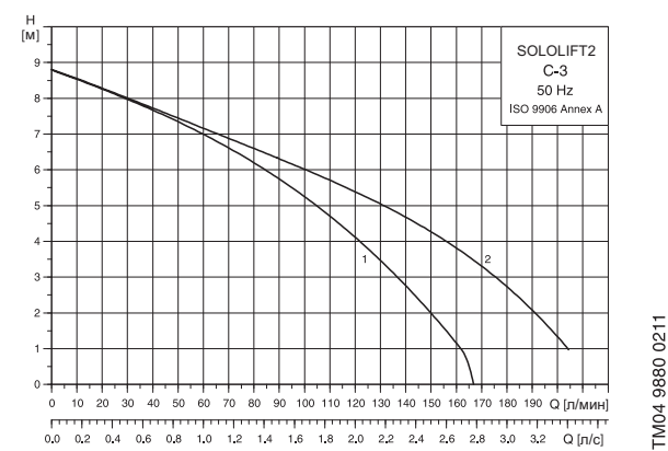
Рис. 65 Кривые характеристик
