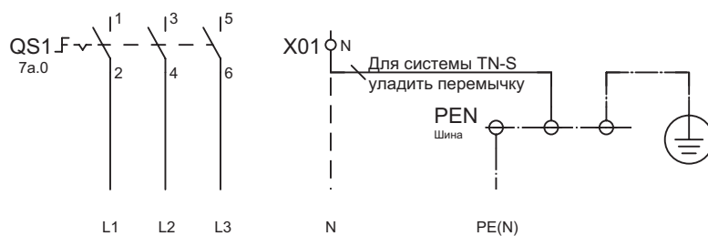
Сеть электропитания
