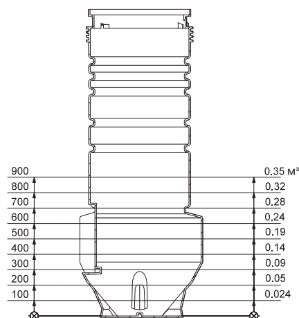
Рис. 138 Полезный объем относительно уровня, PS.R.08
