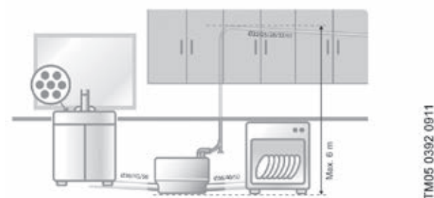
Рис. 53 Для стиральной или посудомоечной машины и кухонной мойки (SOLOLIFT2 C-3)
