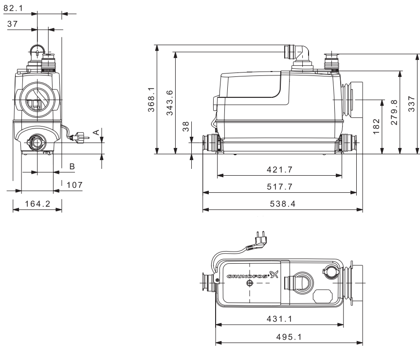
Рис. 63 Габаритные размеры, SOLOLIFT2 CWC-3
