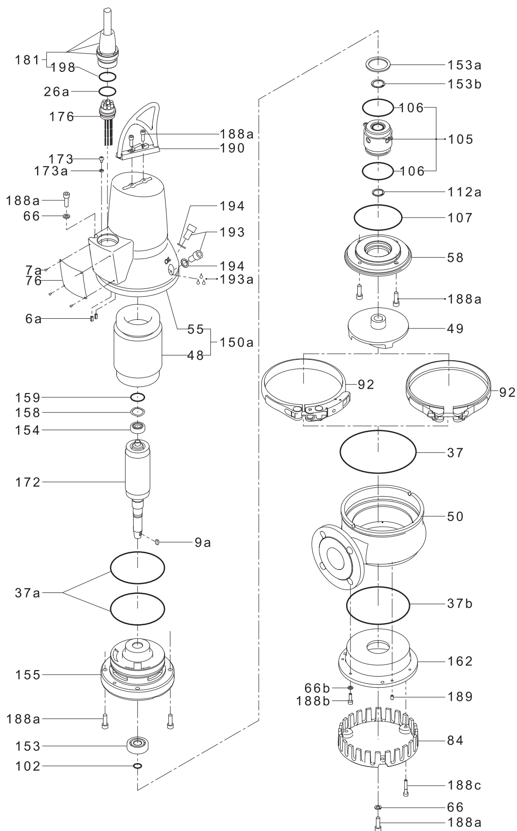
Рис. 11 Деталировка, DP10.65.26
