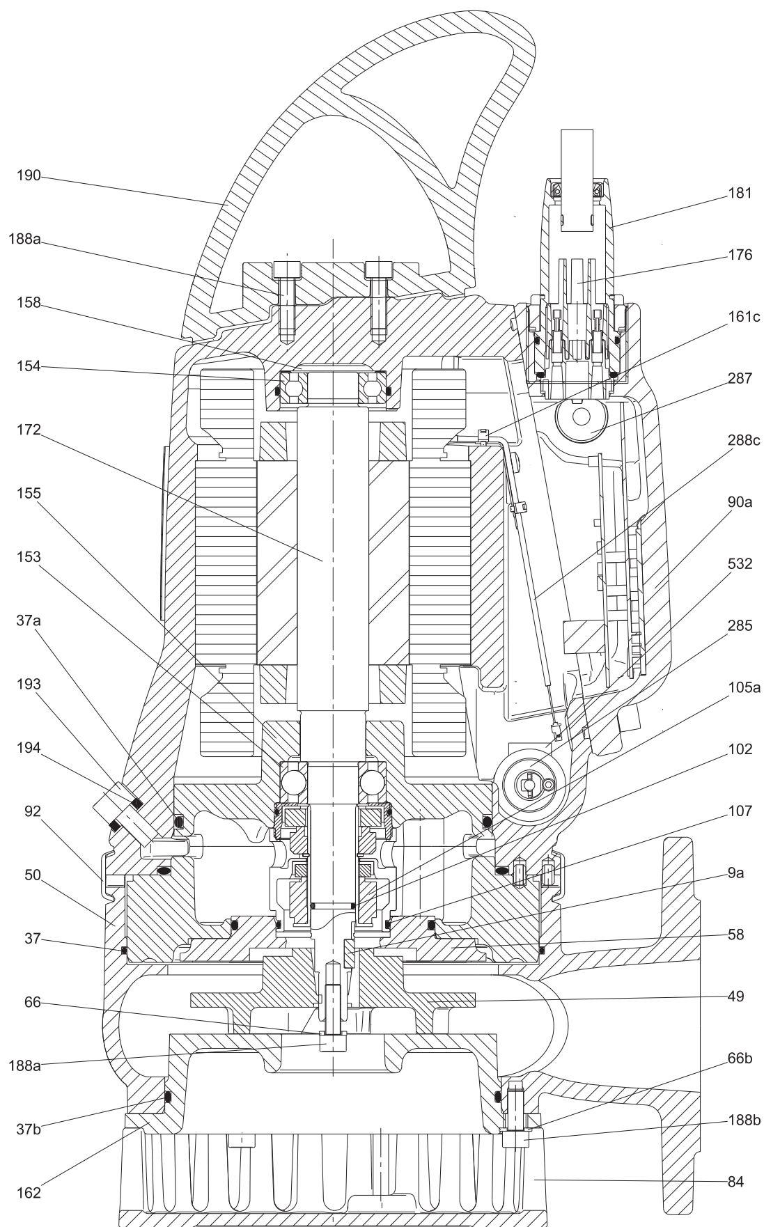
Рис. 16 Чертеж в разрезе, DP10.65.26 AUTO ADAPT
