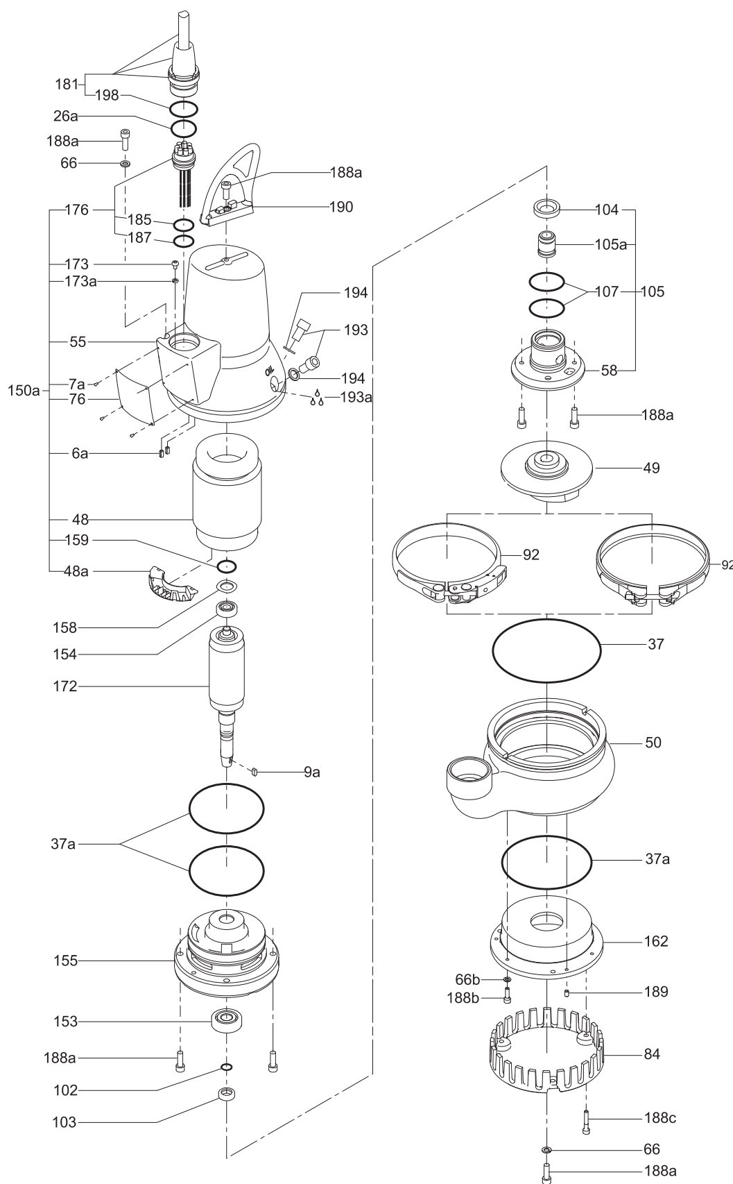
Рис. 9 Детализировка, DP10.50.09/15
