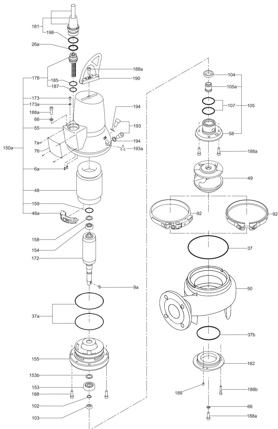
Рис. 21 Деталировка, SL1.50.65.09/11/15
