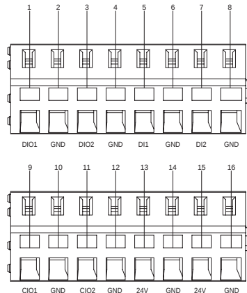
Рис. 53 Клеммы входов/выходов
