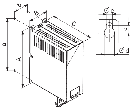
Рис. 148 Настенный монтаж
