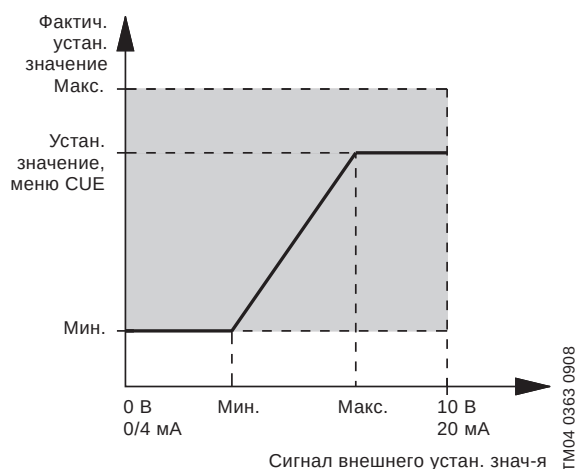
Рис. 110 Сокращённый сигнал внешнего установленного значения
