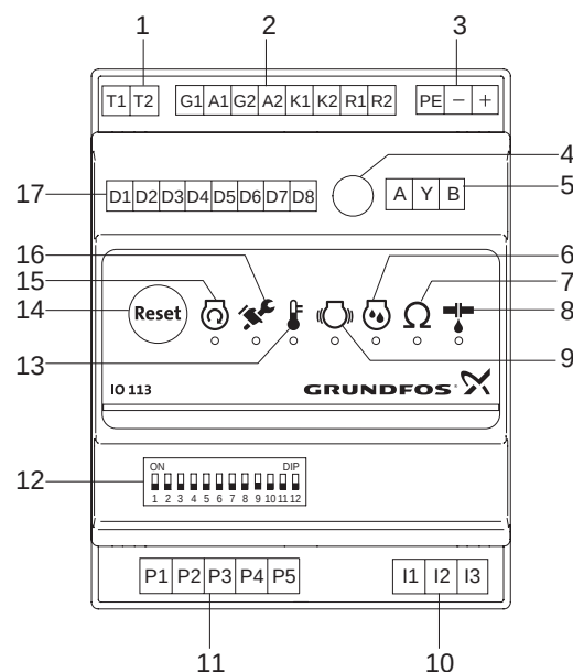
Рис. 163 Модуль IO 113
