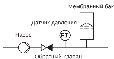
Рис. 96 Расположение обратного клапана и датчика давления в системе, имеющей подпор на входе
