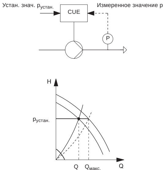
Рис. 115 Регулирование по постоянному давлению
