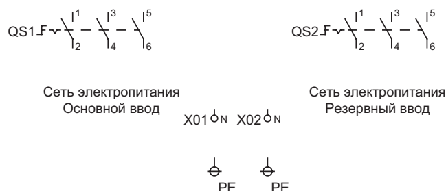
Рис. 43 Двойной ввод питания 3х380V, N, PE с АВР
