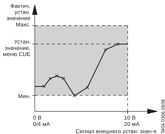
Рис. 114 Внешнее установленное значение по справочной таблице
