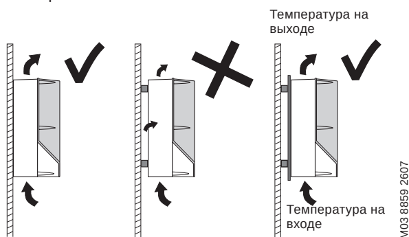
Рис. 135 Вешайте CUE непосредственно на стену или устанавливайте на крепежную пластину с проставками
