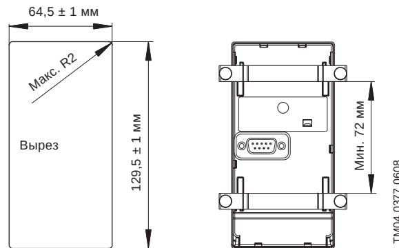
Рис. 155 Монтаж шкафа, размеры выреза
