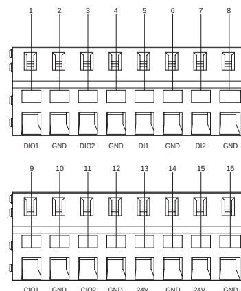
Рис. 10 Клеммы входов/выходов
