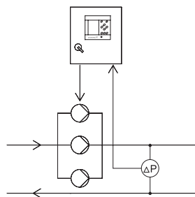
Рис. 22 Перепад давления
