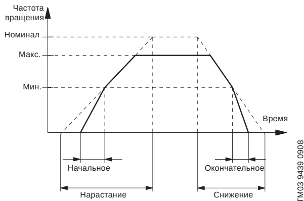
Рис. 128 Нарастание и снижение CUE
