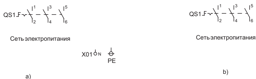
Рис. 42 Один ввод питания: а) 3х380V, N, PE для шкафов с общим потребляемым током до 55 А; б) 3х380V, PE для шкафов с общим потребляемым током более 55 А
