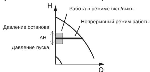
Рис. 94 Постоянное давление с функцией останова. Разница между значениями давления пуска и останова ( \Delta H )
