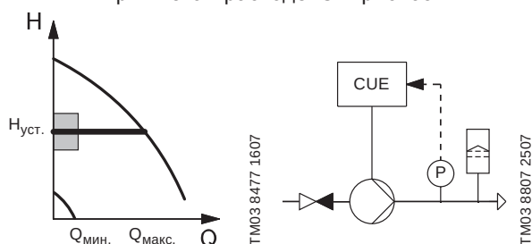
Рис. 93 Постоянное давление с функцией останова
