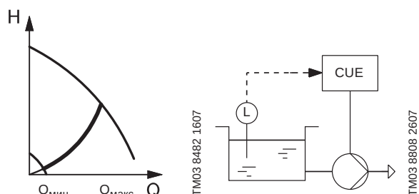
Рис. 104 Постоянный уровень
