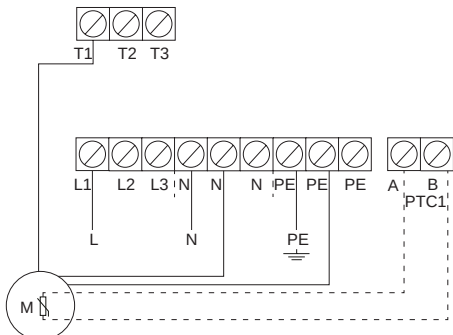
Рис. 48 Однофазное подключение для одного насоса
