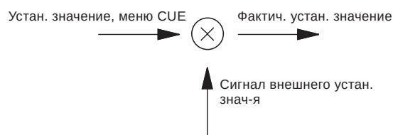
Рис. 108 Установленное значение, меню CUE и сигнал внешнего установленного значения
