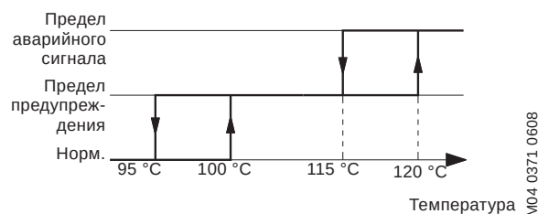
Рис. 133 Контроль температуры подшипников с использованием предельных значений для предупреждений и аварийных сигналов
