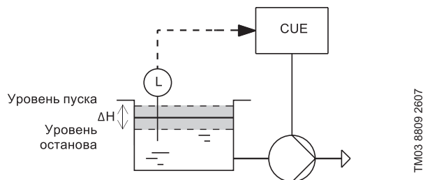
Рис. 106 Постоянный уровень с функцией останова. Разница между уровнями пуска и останова ( \Delta H )
