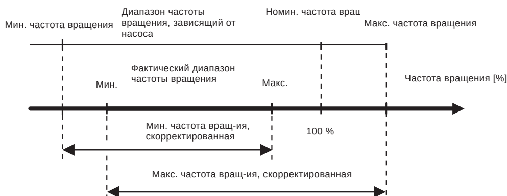
Рис. 129 Установка минимальных и максимальных кривых характеристик в процентах от максимальной производительности.
