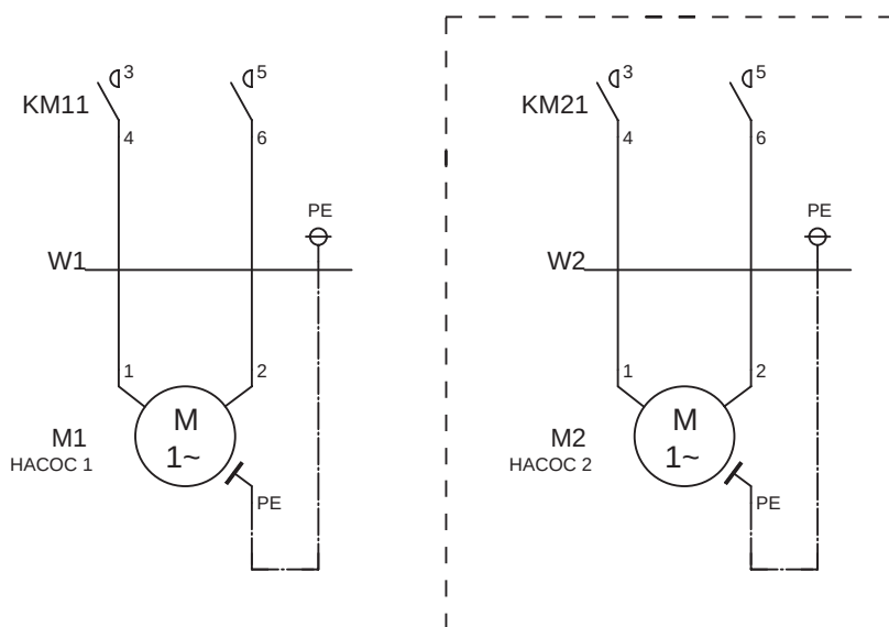
Рис. 55 Подключение однофазных насосов с конденсаторами
