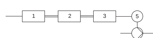
Рис. 141 Погружной насос с соединительной коробкой и экранированным кабелем. Преобразователь частоты и фильтр установлены на большом расстоянии от колодца.
