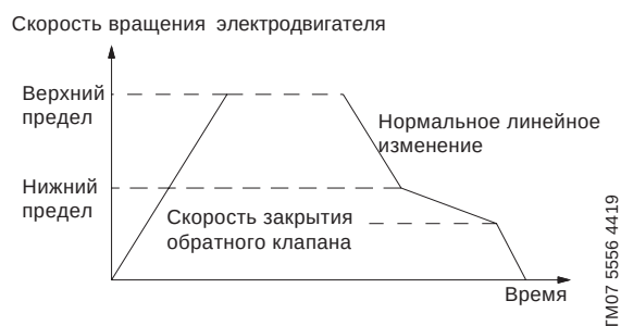
Рис. 132 Контроль скорости закрывания обратного клапана
