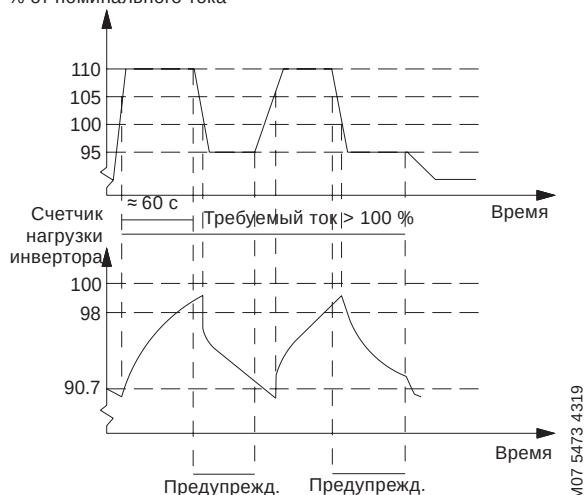
Рис. 123 Выходной ток в условиях перегрузки
