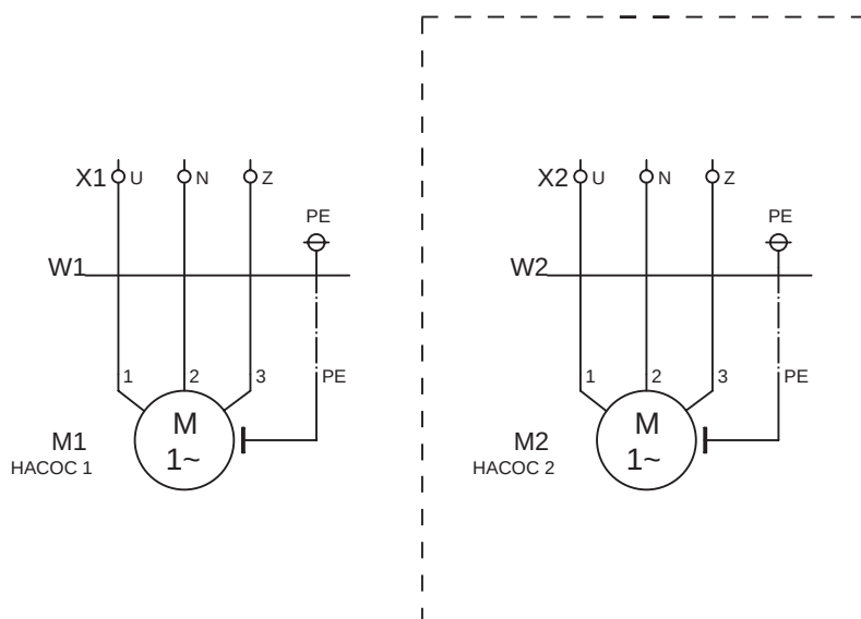
Рис. 56 Подключение однофазных насосов без конденсаторов (конденсаторы в составе шкафа)
