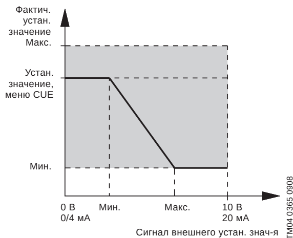
Рис. 112 Сокращённый обратный сигнал внешнего установленного значения.
