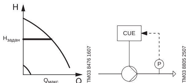
Рис. 92 Постоянное давление
