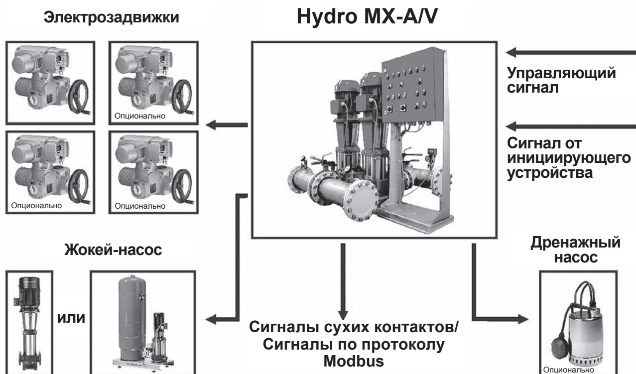
Рис. 83 Общая схема входящих и исходящих подключений
