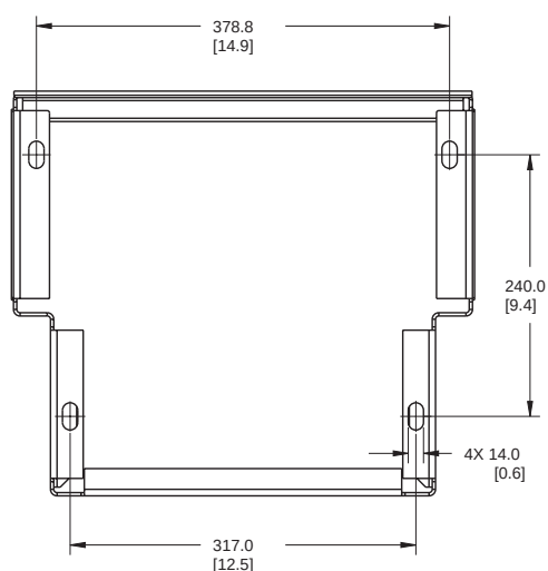
Рис. 157 Шаблон для сверления под цоколь D2h (мм)
