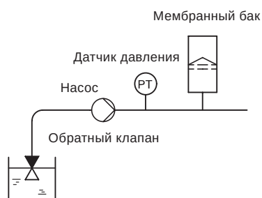
Рис. 95 Расположение обратного клапана и датчика давления в системе, предусматривающей всасывание или работу с отрицательным давлением на входе
