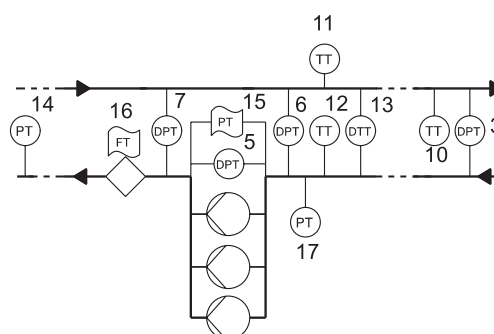
Рис. 31 Отопление и охлаждение, насосы в обратном трубопроводе
