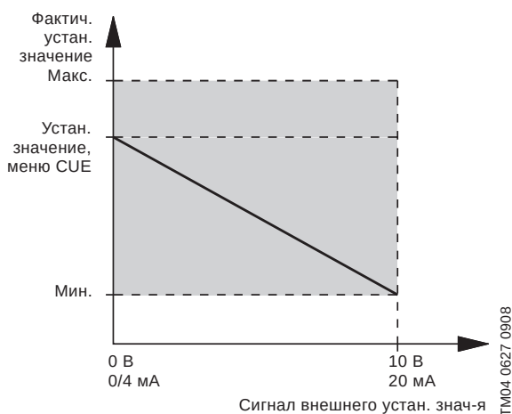
Рис. 111 Обратный сигнал внешнего установленного значения
