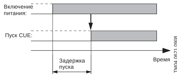
Рис. 124 Задержка пуска после включения питания
