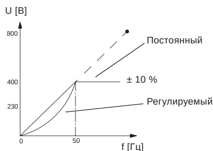
Рис. 121 Регулирование по характеристике U/f (идеальное)
