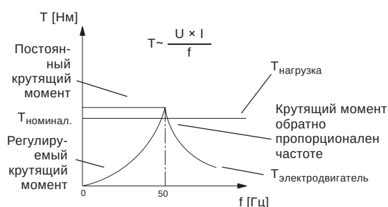
Рис. 122 Регулирование по характеристике T/п (идеальное)
