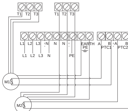
Рис. 51 Трехфазное подключение для двух насосов
