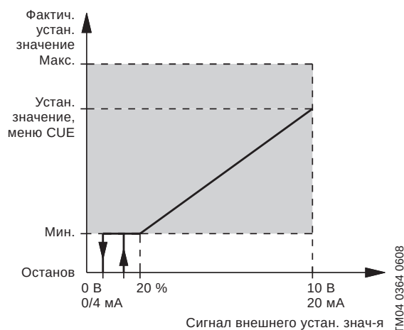
Рис. 113 Внешнее установленное значение с функцией останова
