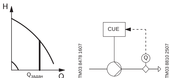
Рис. 103 Постоянный расход
