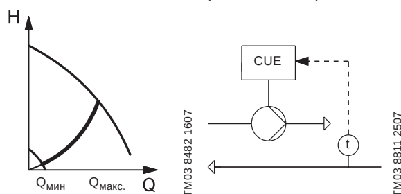
Рис. 107 Постоянная температура
