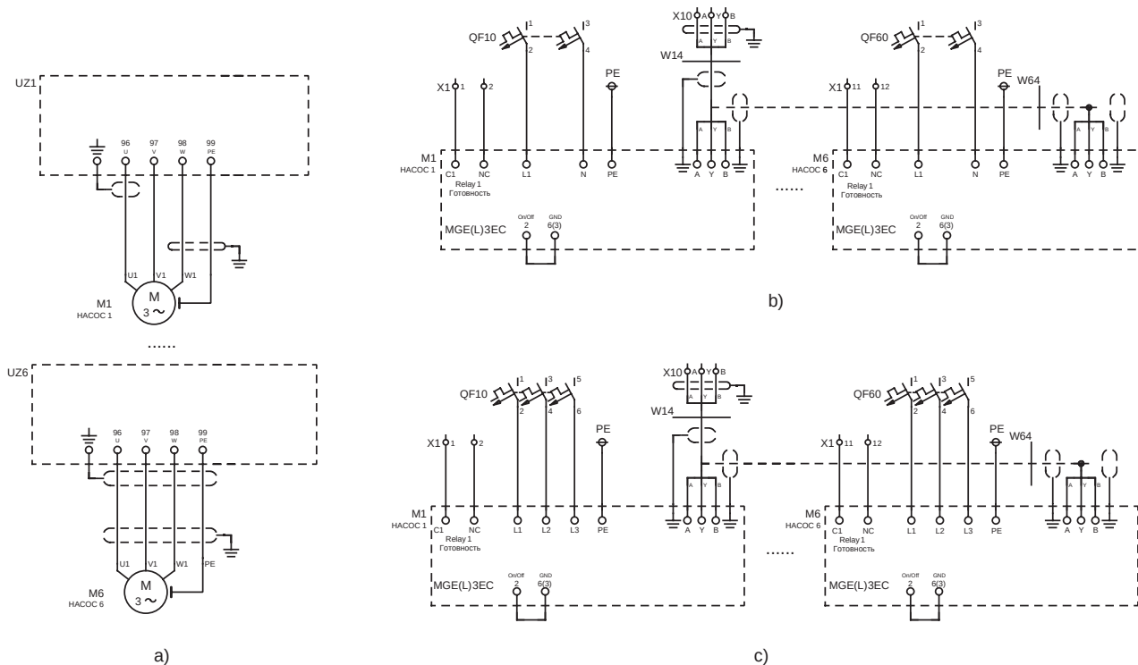
Рис. 45 Подключение насосов по схеме: а) через преобразователи частоты в шкафу (ESS); б) через преобразователи частоты на насосах 1х220В; в) через преобразователи частоты на насосах 3х380 В
