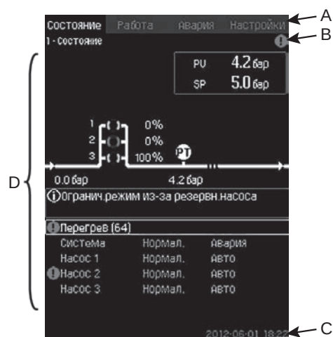
Рис. 19 Структура дисплея
