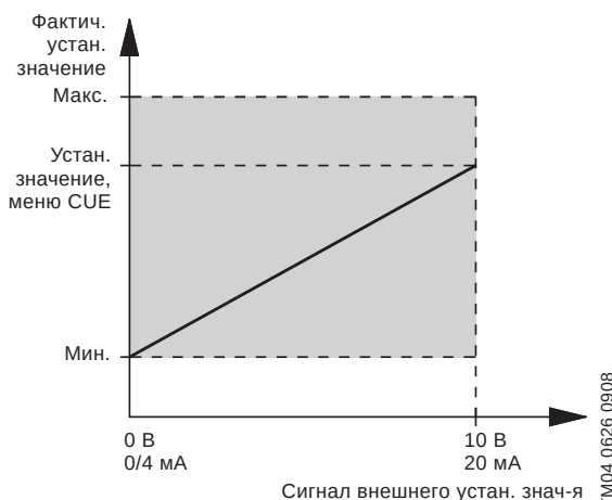
Рис. 109 Внешнее установленное значение
