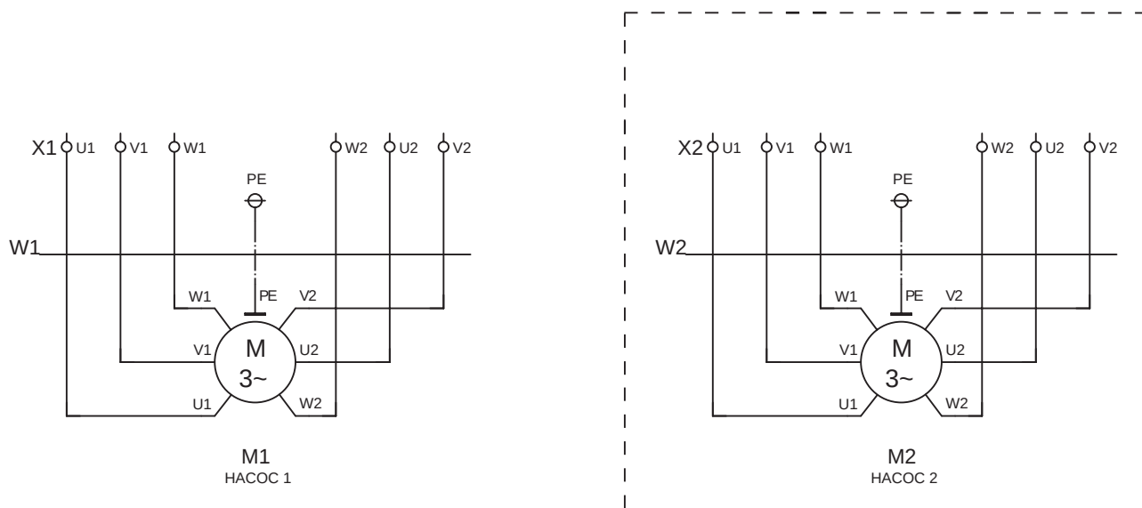
Рис. 59 Подключение трёхфазных насосов по схеме «звезда-треугольник» (SD)
