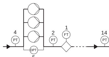
Рис. 29 Повышение давления
