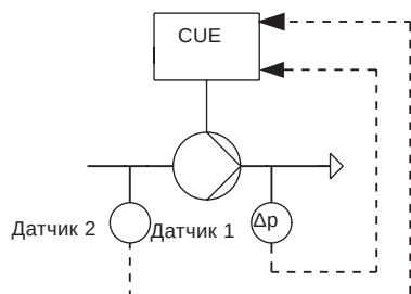
Рис. 99 Перепад давления от двух датчиков
